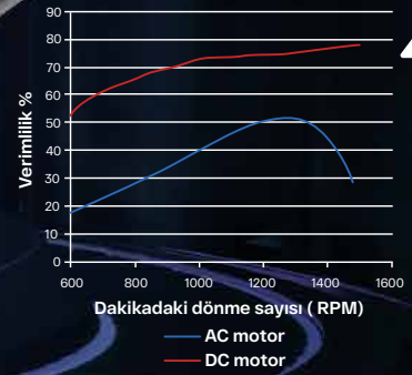
AC ve DC motor verimlilik karşılaştırma
